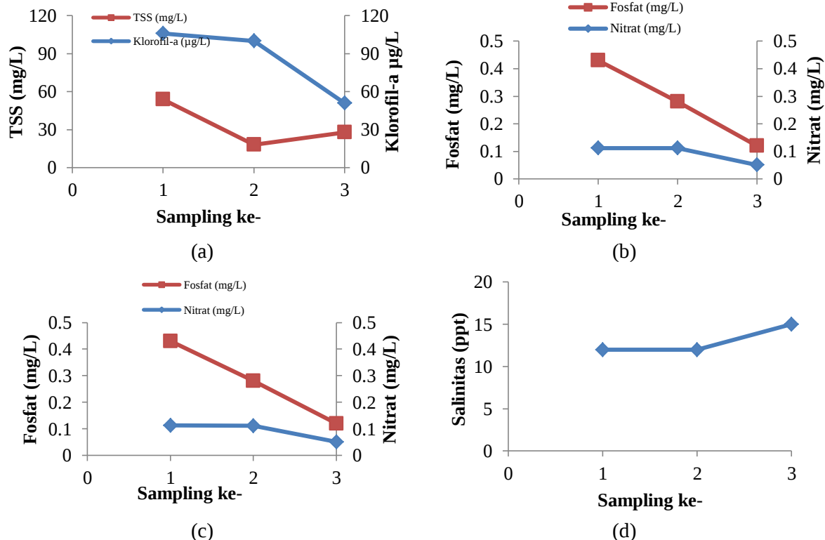
Gambar 3. (a) TSS & Klorofil-a (b) Kecepatan arus & Kecerahan (c) Nitrat & Fosfat (d) Salinitas di Stasiun 1
