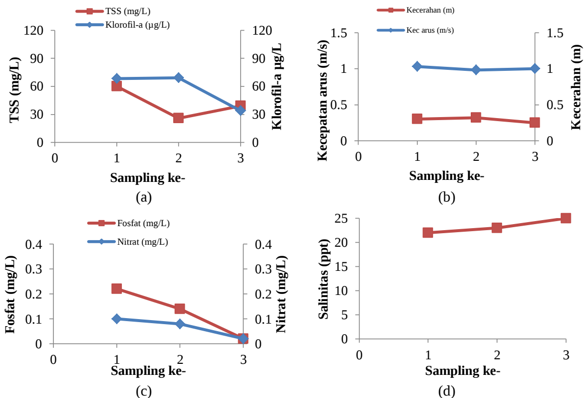
Gambar 4. (a) TSS & Klorofil-a (b) Kecepatan arus & Kecerahan (c) Nitrat & Fosfat (d) Salinitas di Stasiun 2
