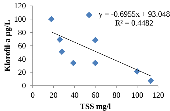
Gambar 6. Hubungan TSS dan Klorofil-a
