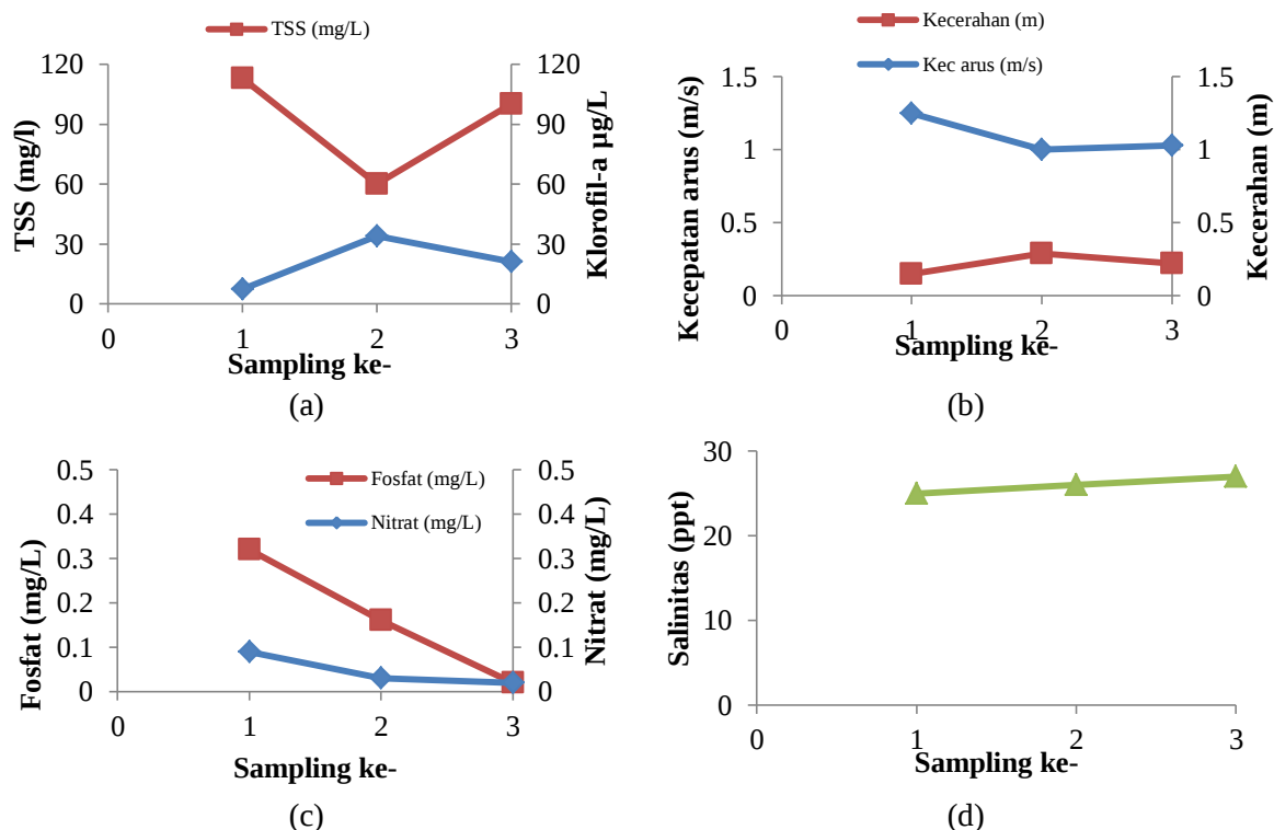
Gambar 5. (a) TSS & Klorofil-a (b) Kecepatan arus & Keccerahan (c) Nitrat & Fosfat (d) Salinitas di Stasiun 3
